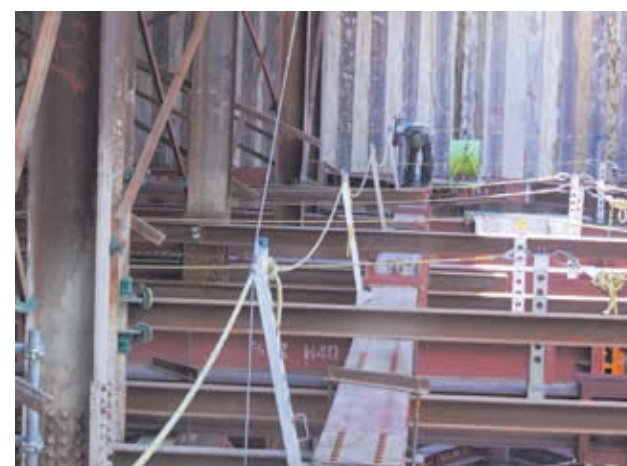
鉄骨用親綱支柱 SUPER-301
