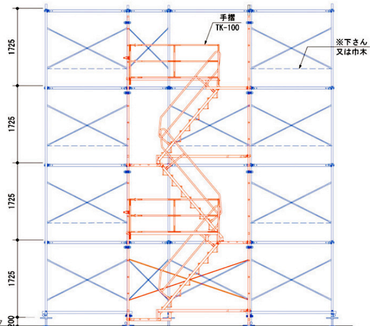
A-A立面図
