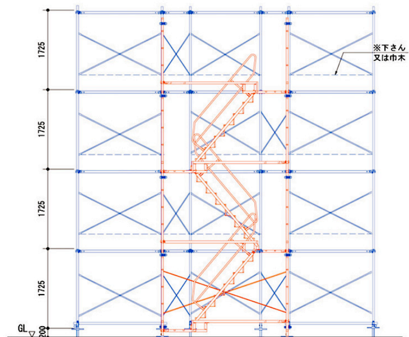
A-A立面図
