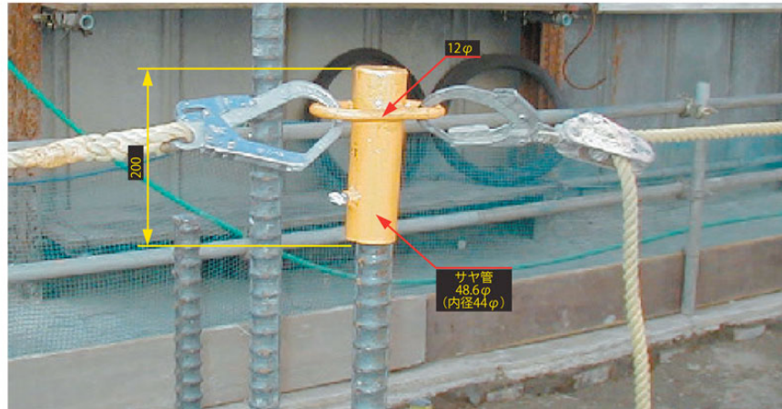
親網用鉄筋キャップ G-201T 重量(1.5kg)
