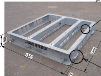
&lt;段差通路用架台 G-200H&gt;
