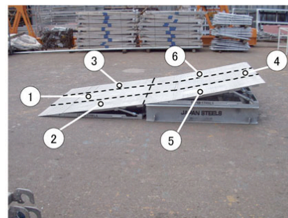
&lt;高さ調整&gt;
