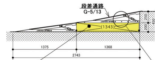
&lt;上側段差通路取付&gt;
