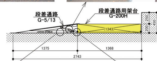
&lt;下側段差通路取付&gt;
