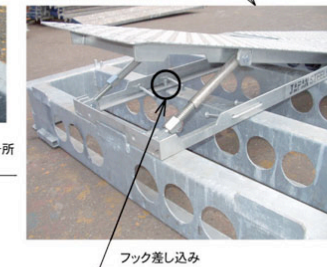
フック差し込み
