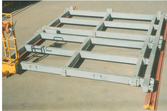
本体 RP-30/20
