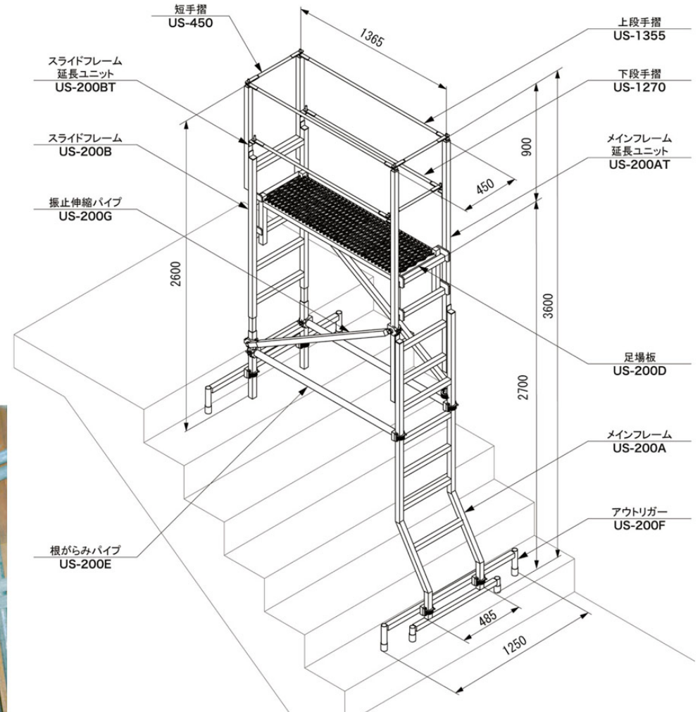
ヤングマン「延長タイプ」 H = 2700型
