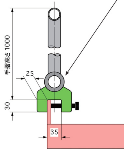
クランプ部詳細
