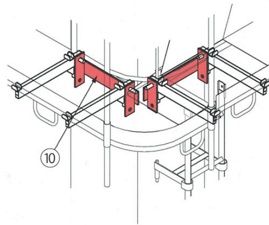
先付けピース部詳細
