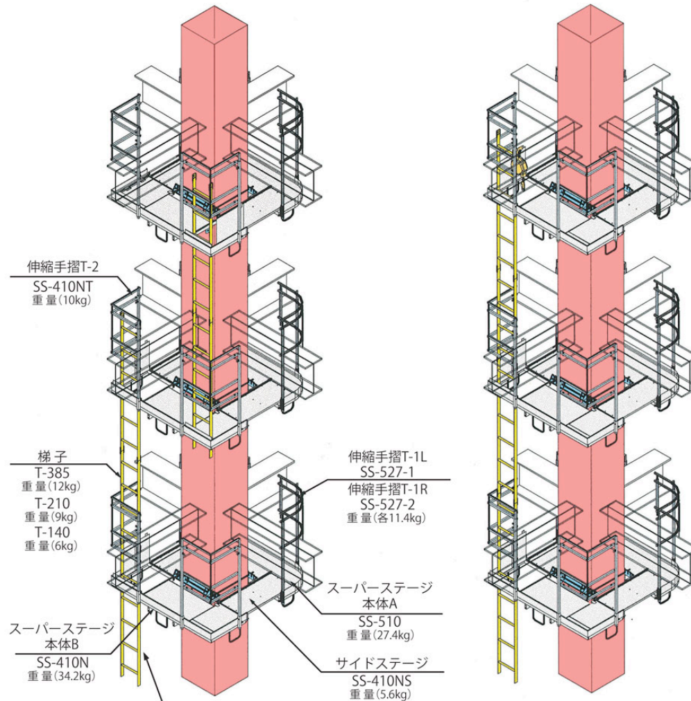
梯子取付パターンA
